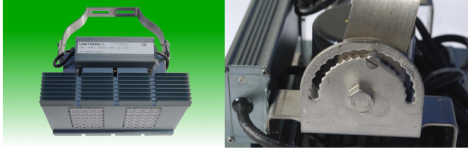
UDL2 Aufputzmontage (AP):
